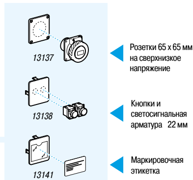
Щитки для промышленных разъёмов
