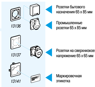
Щитки для модульных устройств с интерфейсным модулем и интерфейсные модули
